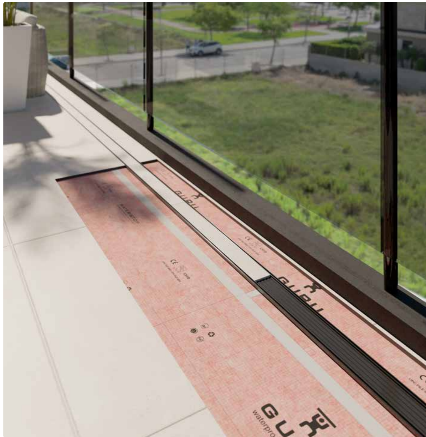
Canal y rejilla RAYNEX de doble ranura con impermeabilización.
