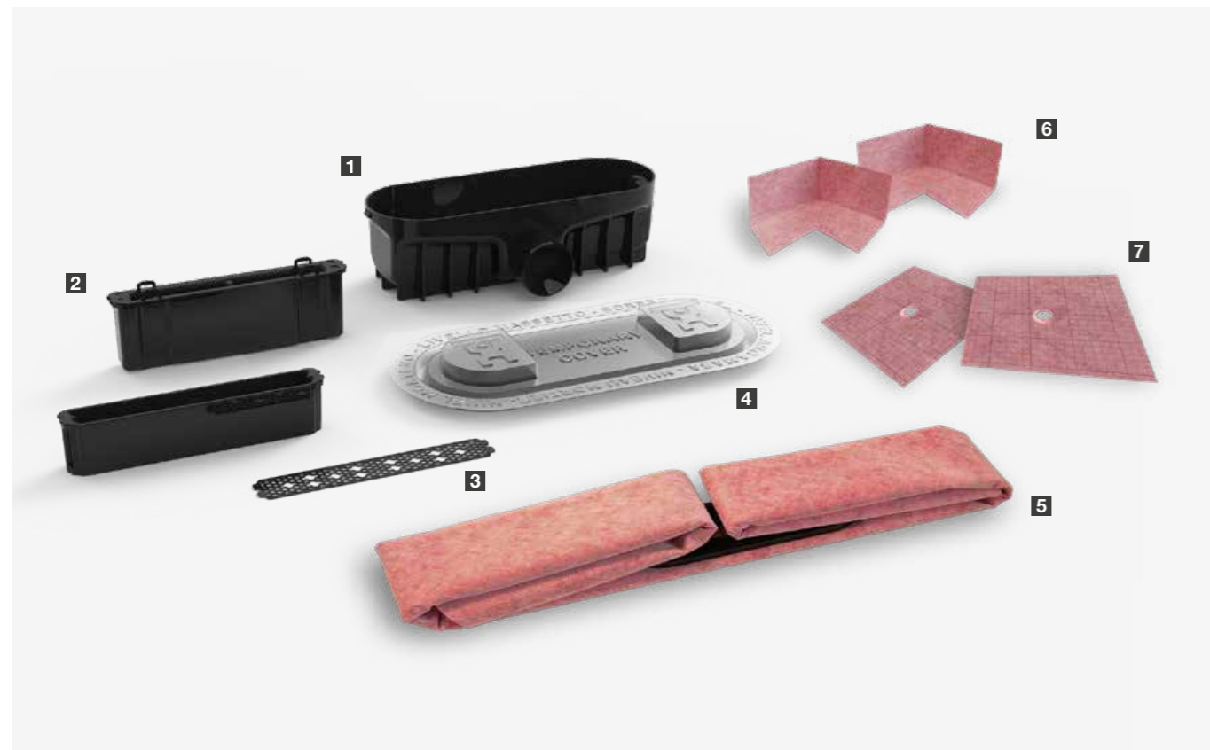
1- Sumidero a elegir (TRYPHON, TRYPHON REDUCIDO o TRYPHON VERTICAL). 2- Sifón intercambiable (hidráulico y seco). 3- Recogepelos. 4- Tapa de nivel de mortero. 5- Lámina WATER-STOP con adaptador termosellado. 6- W-S DIN x2 (esquina interior). 7- W-S TUB x2 (tuberías pasantes).
