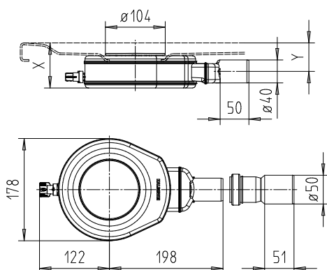
KA 90 PLANO
