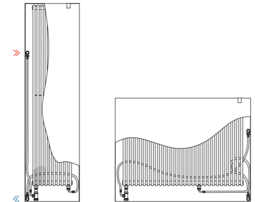
Figura 3A (Cód. L1 / L2 / L3 / L4 / L5) SISTEMA DE CONEXIÓN HIDRÁULICA OCULTO Sin incremento de precio.
